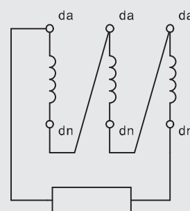
电压继电器 Voltage relay
