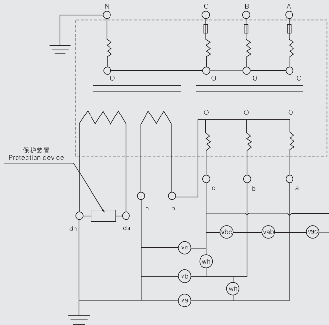
双计量接线原理图
